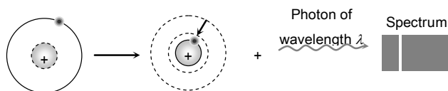
Fig. 26.9 : Emission spectra
